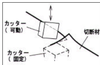
刃部構造図
