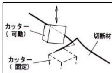
刃部構造図
