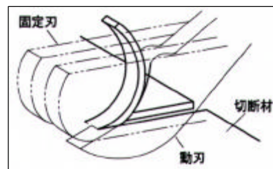
刃部 構造図
